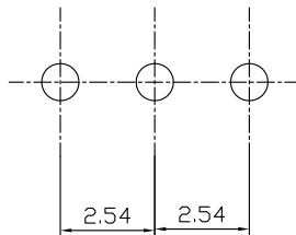
P.C.B DIMENSION
